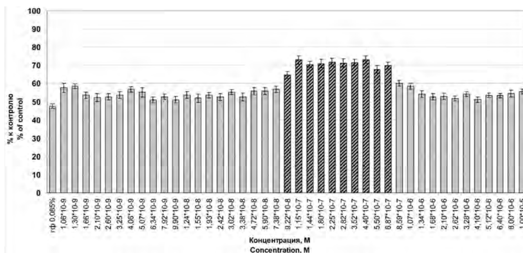
Рис. 4. Зависимость длины корня от концентрации БС у сорта льна-долгунца Веста, при концентрации глифосата 0,085 %, выраженная в процентном отношении к контролю (1 % Гисинар)
