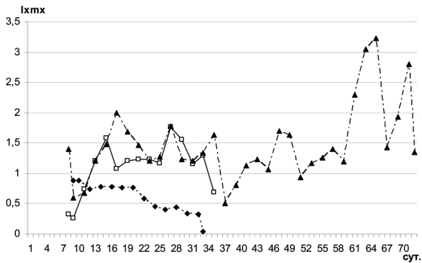
Рис. 2. Средневзвешенная, относительно выживаемости, плодовитость D. longispina при разных концентрациях пищи: \blacklozenge – 0,08; \square – 0,18; \blacktriangle – 0,36 мг/л
