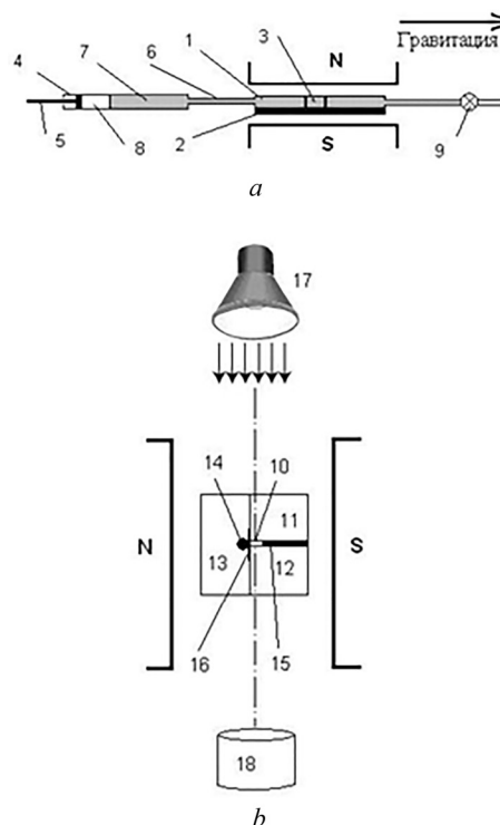
Рис. 1. Схема микрожидкостной системы (а) и магнитофоретической измерительной ячейки (б) магнитоцитометра [8]: 1 – измерительная ячейка; 2, 14 – ферромагнитный стержень; 3 – область регистрации; 4 – микрошприц; 5 – поршень; 6 – игла; 7 – исследуемая клеточная суспензия; 8 – воздух; 9 – клапан; 10 – щелевой канал; 11–13 – детали из оптического стекла К-8; 15, 16 – вставки из алюминиевой фольги; 17 – светодиодная подсветка; 18 – объектив USB микроскопа; N, S – полюса магнита
