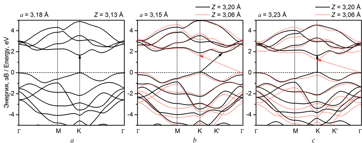
Рис. 2. Электронная зонная структура монослоя \text{MoS}_2 с недеформированной ( a ) и деформированной ( b , c ) кристаллической решеткой. Ноль на шкале энергии соответствует положению максимума валентной зоны
